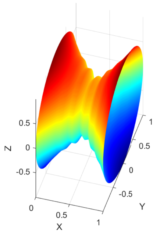
Sólido de revolución ( n=15 , t_k=0.15 )
